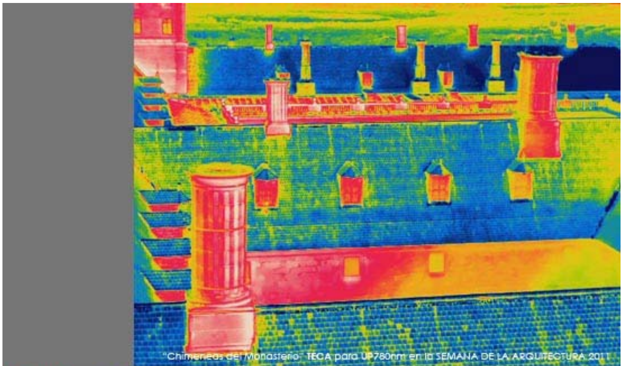
CHIMENEAS. TERMOGRAFÍA. 550 X 325 Puntos a 72ppp en RGB. SEPTIEMBRE 2011.
